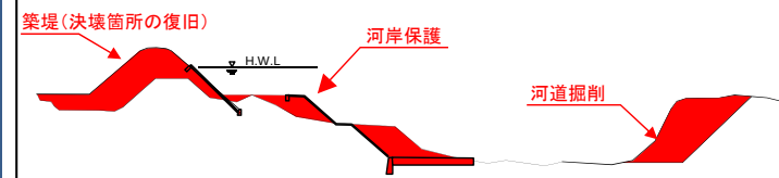
災害復旧、関連事業イメージ
